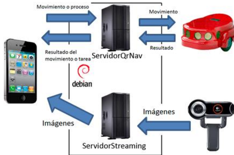
Figura 9 - Estructura paso de mensajes
