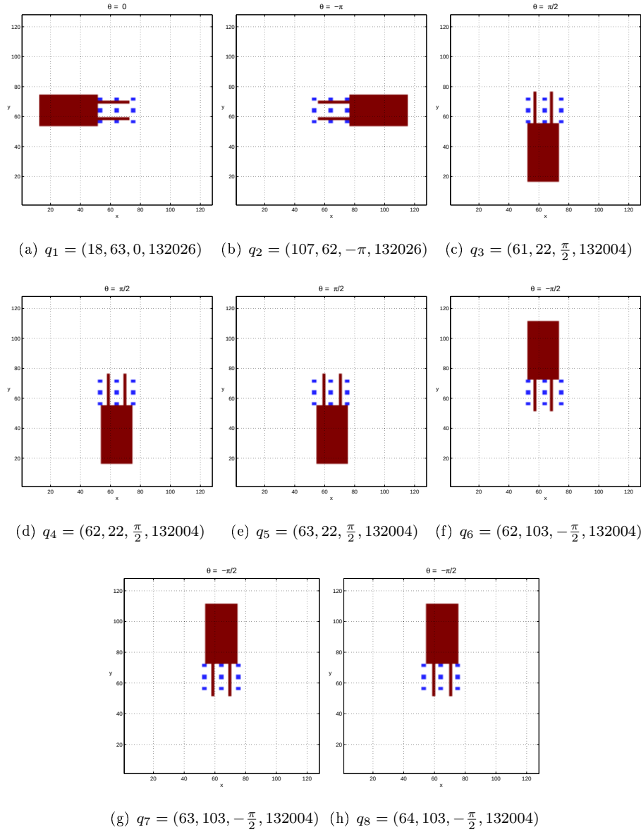
Figura 5.7: Robot en las configuraciones de agarre con zona de agarre en la horquilla del robot y en los tacos centrales del palé.
