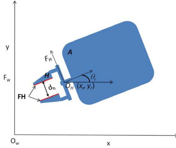
Figura 3.4: Robot rígido con pinzas paralelas que se desplaza y gira libremente.
