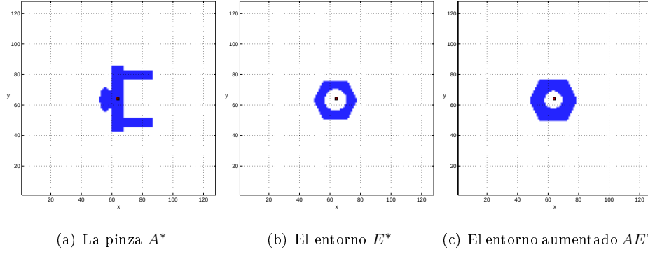
Figura 4.3: Discretización de las funciones para el escenario básico con resolución N = 128 .
