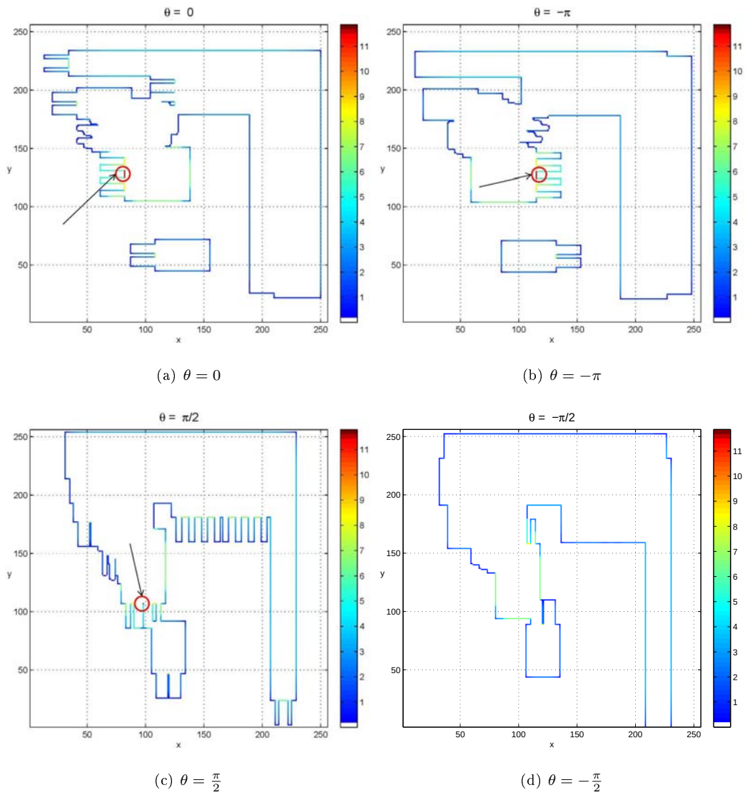
Figura 5.13: Frontera de agarre en las orientaciones 0 , -\pi y \frac{\pi}{2} donde se producen los agarres y en -\frac{\pi}{2} donde no es posible agarrar el objeto.
