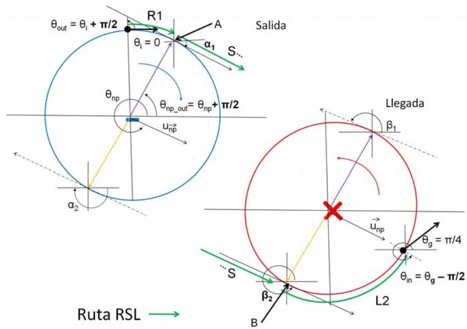
Figura A.3: Esquema del cálculo de la curva de Dubins RSL.
