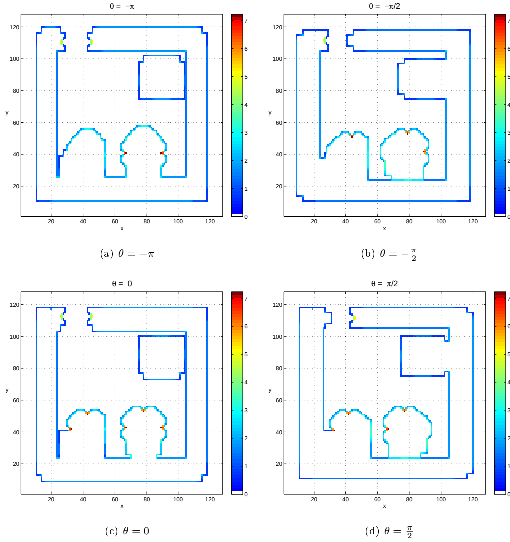
Figura 4.44: Frontera de agarre en 2D del escenario de la figura 4.38 en las orientaciones donde se obtienen las configuraciones de los mejores agarres.
