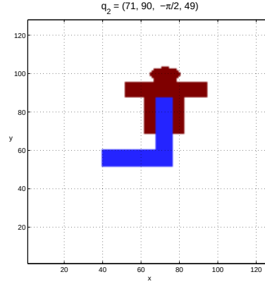
Figura 4.10: Configuración de agarre para pieza en “L” para pinza con orientación \theta = -\frac{\pi}{2} .
