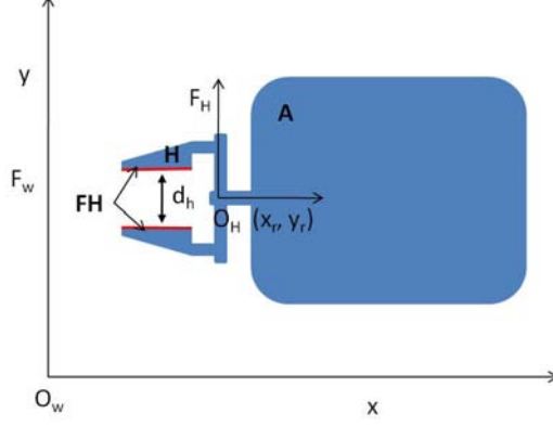
Figura 3.3: Robot r gido con pinzas paralelas.
