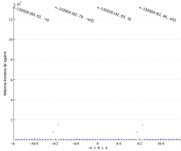
Figura 5.8: Frontera de agarre en todas las orientaciones.
