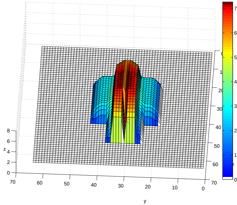
Figura 4.19: Pieza barra vertical proyectada en C .
