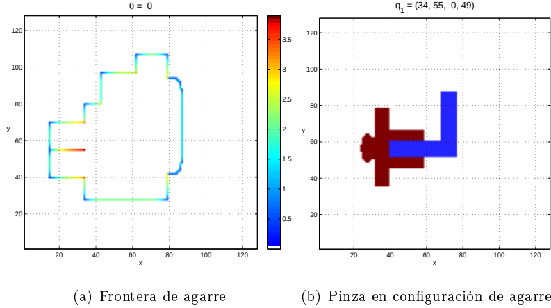
Figura 4.8: Configuración de agarre para pieza con forma de "L"
