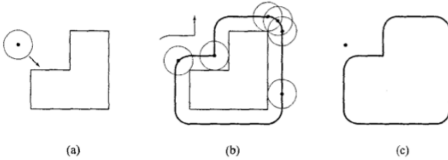
Figura 2.4: Entorno de trabajo y obstáculos.
