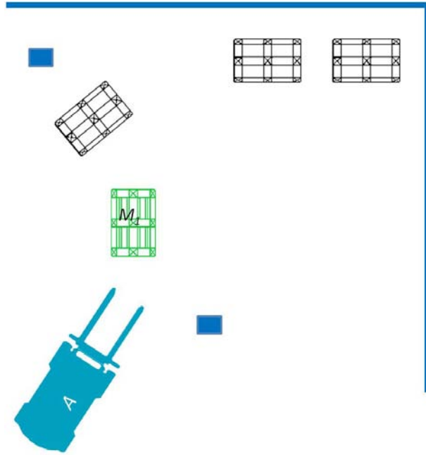
Figura 5.10: Escenario de trabajo del robot paletizador.
