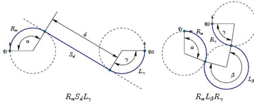
Figura 5.15: Trayectorias de dos de las curvas de Dubins en W = \mathbb{R}^2
