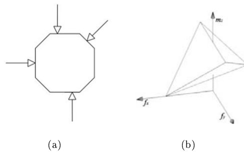
Figura 2.7: No se cumple la condición de force/torque closure .
