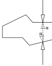
Figura 2.8: Se cumple la condición de force closure en un agarre con dos dedos.
