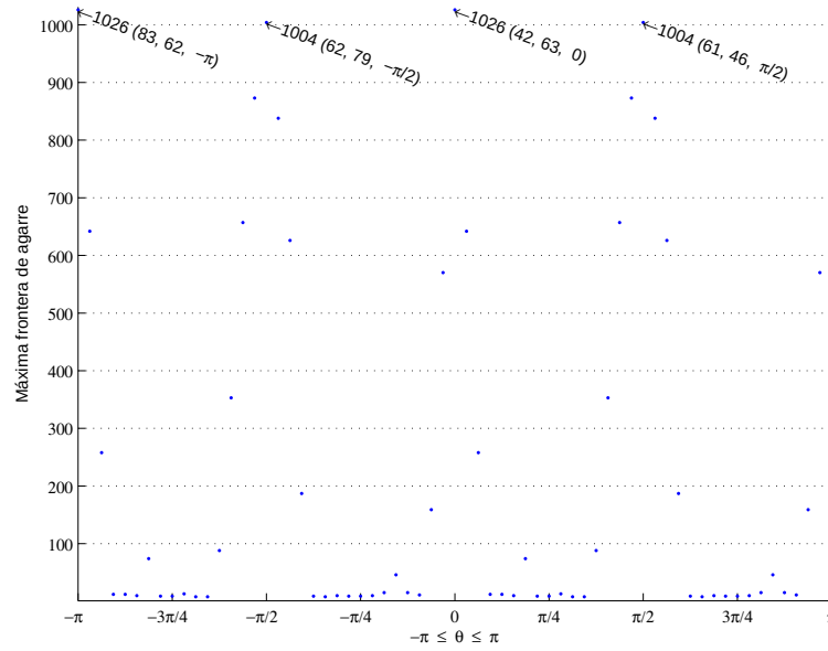
Figura 5.4: Valores máximos de la frontera de agarre para todas las orientaciones.
