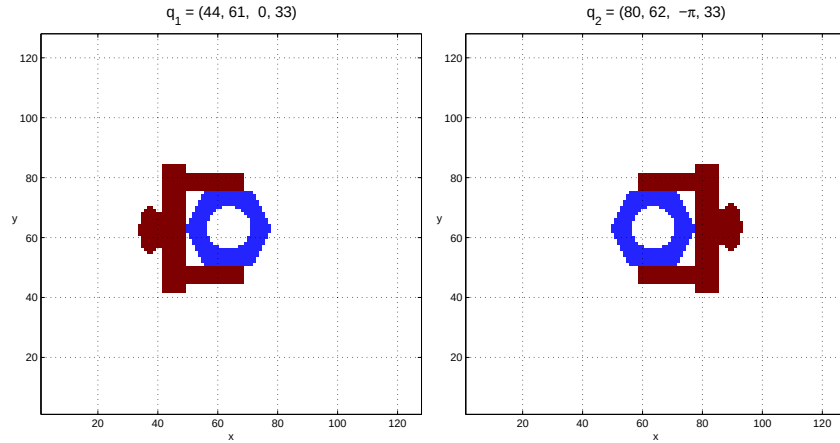
(a) Pinza en la configuración de agarre (44, 61, 0) en W (b) Pinza en la configuración de agarre (80, 62, -\pi ) en W
