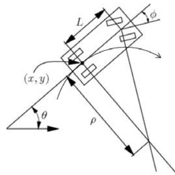
Figura 5.14: El coche sencillo.
