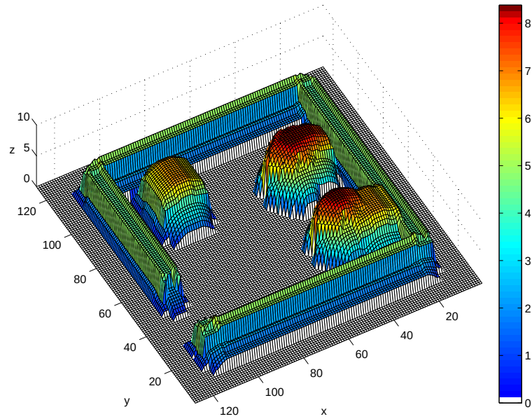
Figura 4.40: C-espacio en la orientación \theta = -\frac{\pi}{2} .
