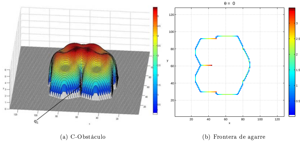
Figura 4.4: Tuerca proyectada en el C-espacio. En z se muestra el logaritmo de la convolución, para mayor claridad. q_1 es la configuración de agarre.
