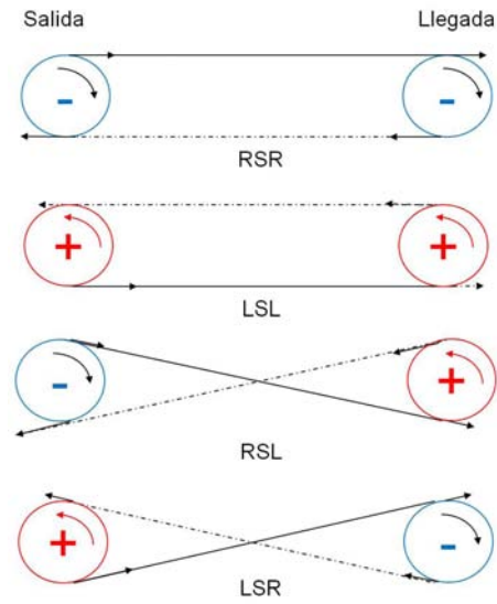
Figura 5.16: Cálculo de las curvas de Dubins.
