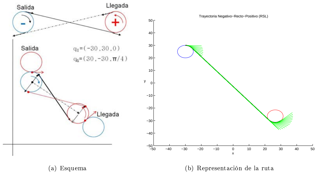
Figura 5.20: Curva de Dubins RSL.
