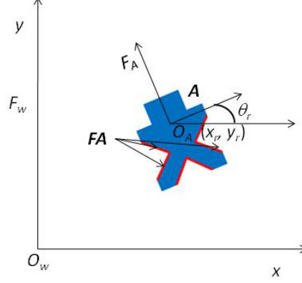
Figura 3.2: Elecci n de los sistemas de referencia.
