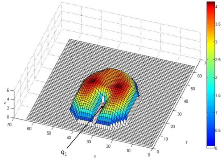
Figura 4.12: Proyección en la pieza en C para el escenario de la figura 4.11. El eje z está en escala logarítmica. q_1 es la configuración de agarre.
