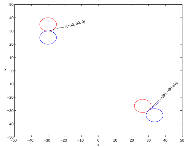
Figura 5.17: Circunferencias con sentido positivo y negativo en la configuración inicial y final.
