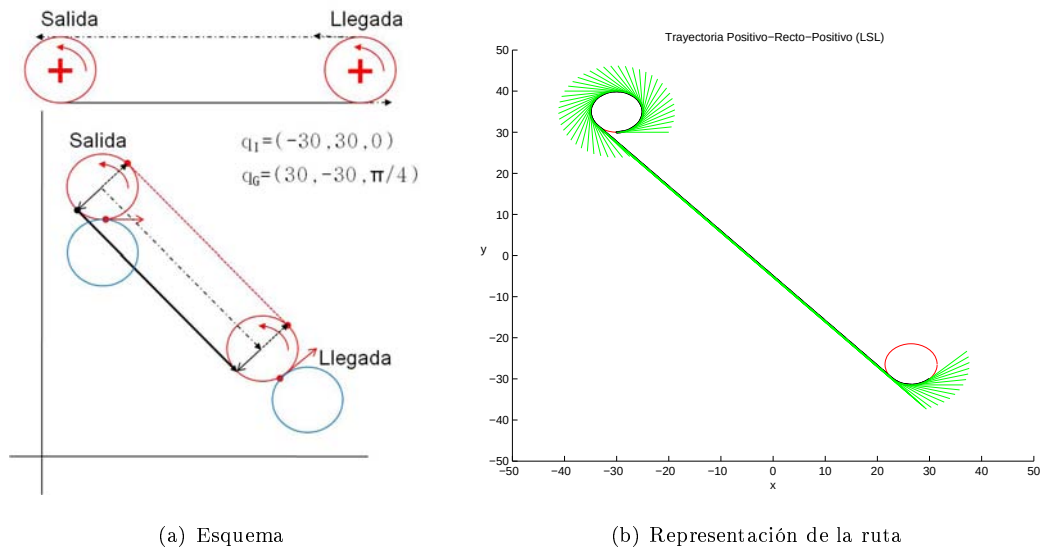
Figura 5.18: Curva de Dubins LSL.
