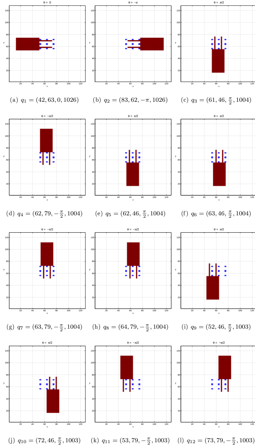
Figura 5.6: Robot en las configuraciones de agarre cuando se especifica únicamente la zona de agarre en su horquilla.
