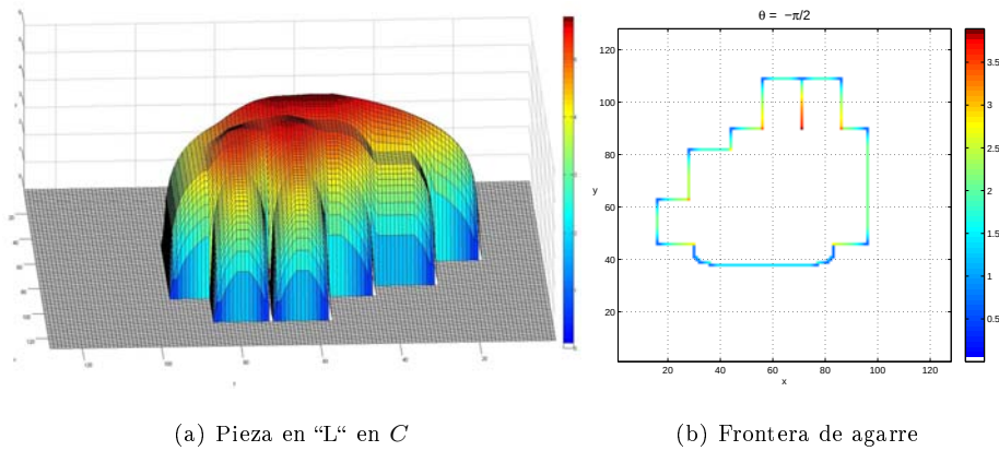
Figura 4.9: Pieza con forma de "L" en C y su frontera de agarre para pinza con orientación \theta = -\frac{\pi}{2}
