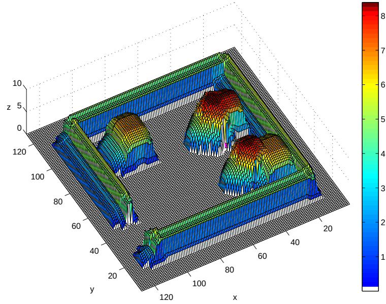
Figura 4.39: C-espacio en la orientación \theta = -\pi .
