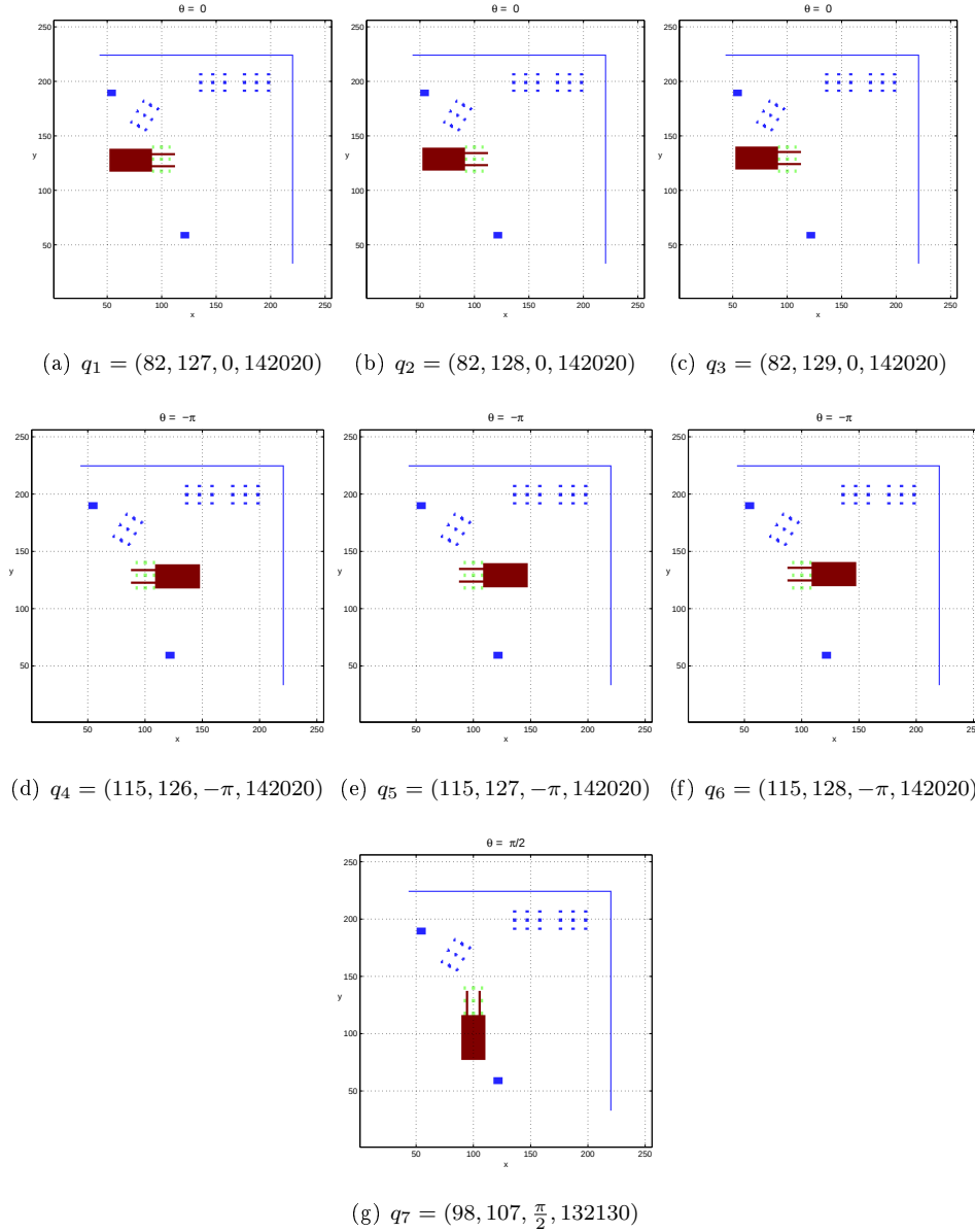
Figura 5.12: Robot en las configuraciones de agarre en un escenario con obstáculos y con objetos movibles.
