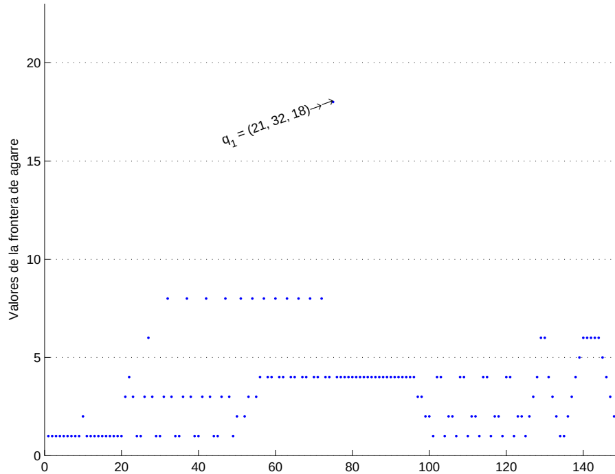
Figura 4.13: Perfil de la frontera de agarre. La configuración de agarre se alcanza en q_1(x, y) = (21, 32) con el valor máximo de 18.
