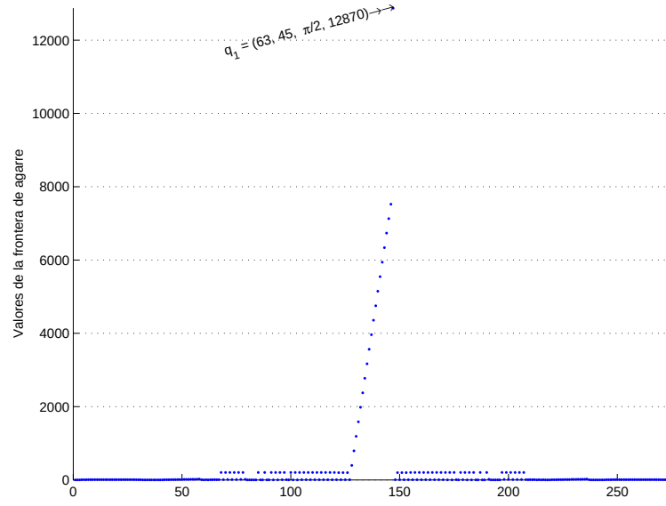
Figura 4.29: Valores de la frontera de agarre para la orientación \theta = \frac{\pi}{2} .
