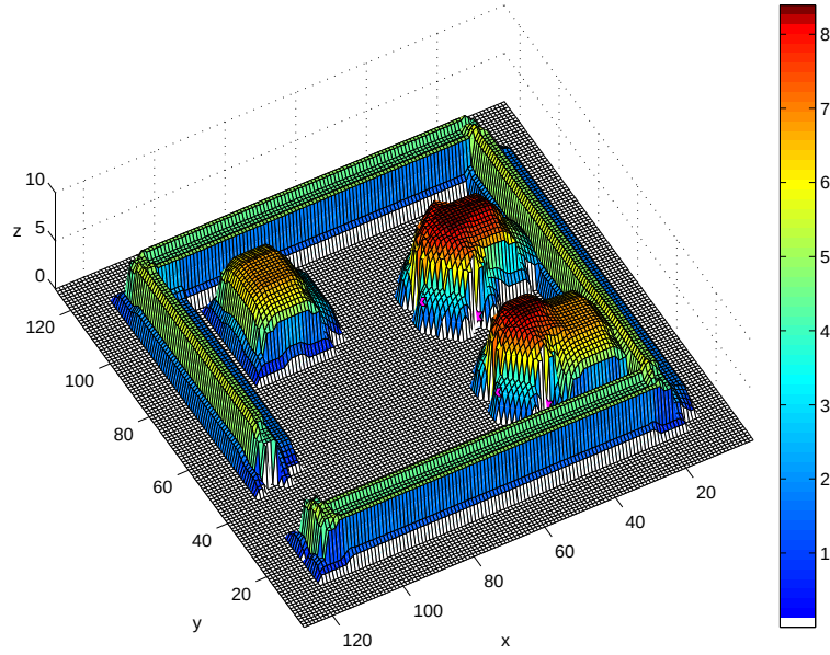
Figura 4.41: C-espacio en la orientación \theta = 0 .
