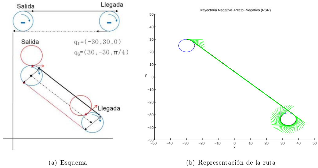
Figura 5.19: Curva de Dubins RSR.
