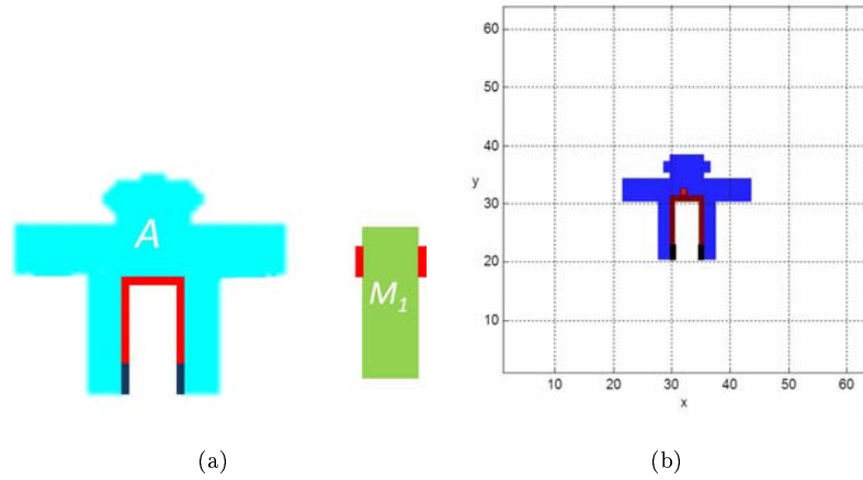
Figura 4.22: Escenario con zonas de agarre en la yema de los dedos de la pinza y en el objeto.
