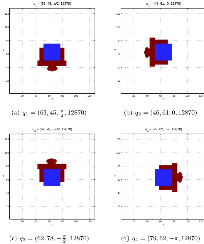
Figura 4.28: Mejores agarres considerando la orientación.
