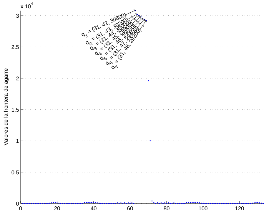
Figura 4.20: Perfil de la frontera de agarre con máximos locales seleccionado con umbral u .
