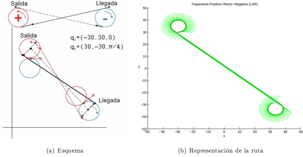
Figura 5.21: Curva de Dubins LSR.
