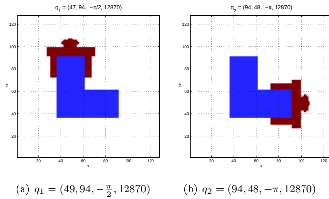
Figura 4.32: Pinza agarrando la pieza en L.
