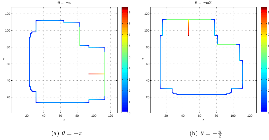
Figura 4.31: Frontera de agarre en 2D en las orientaciones donde se obtienen las configuraciones de los mejores agarres.
