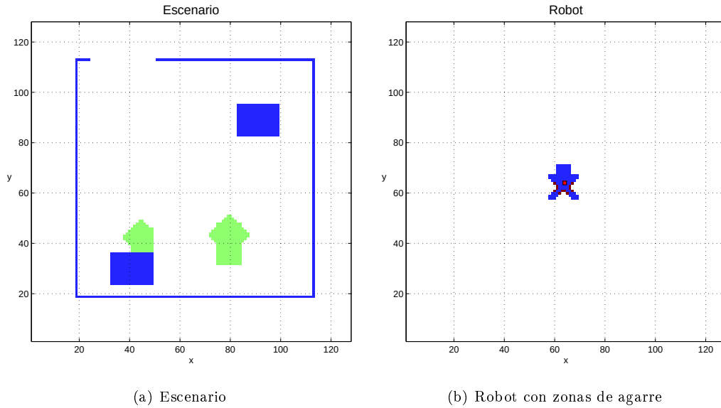
Figura 4.38: Robot con zonas de agarre en un escenario con objetos movibles y obstáculos.
