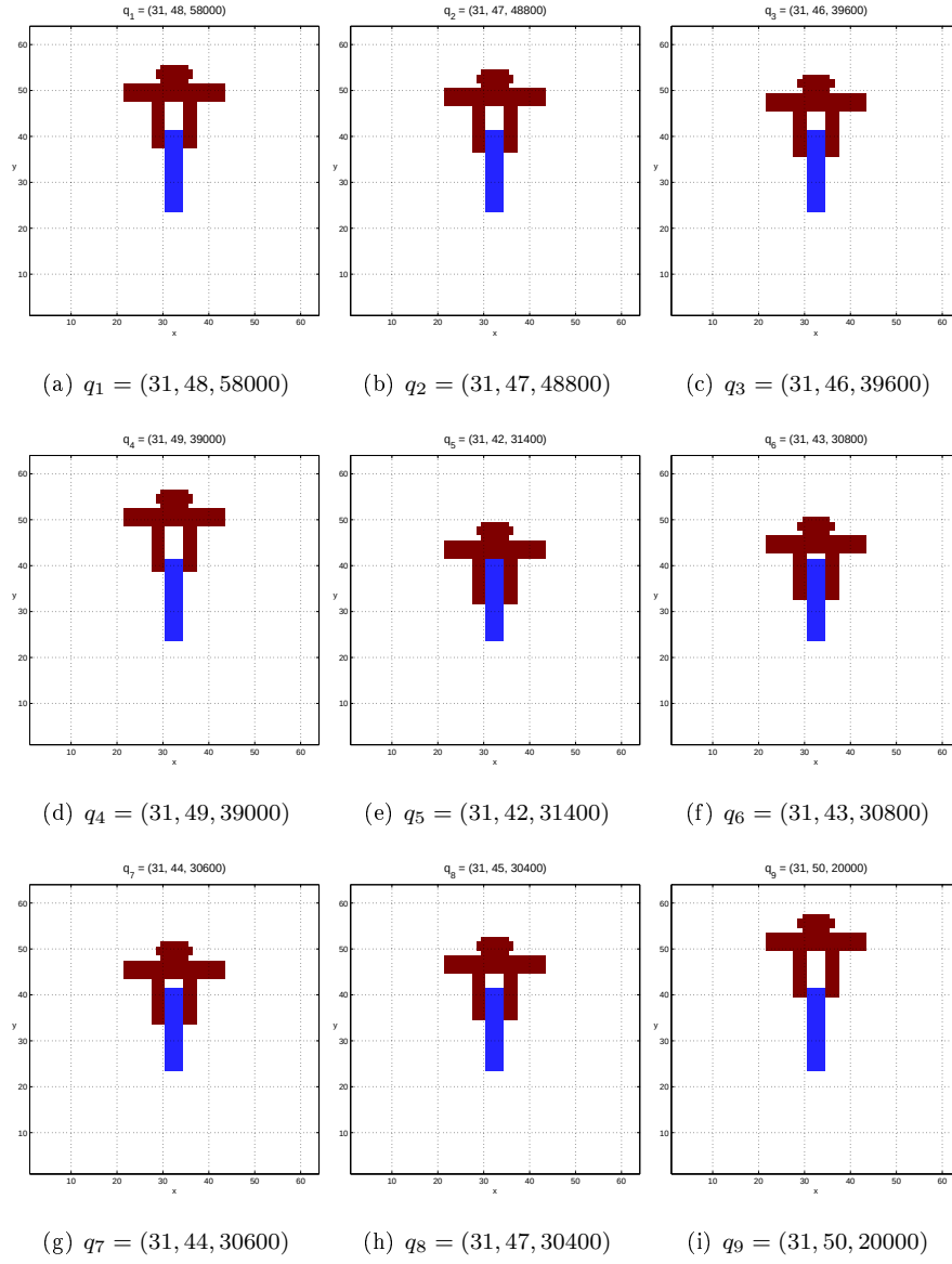
Figura 4.24: Mejores agarres con zona de agarre en el objeto y en la yema de los dedos de la pinza.
