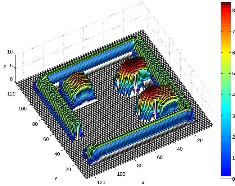
Figura 4.42: C-espacio en la orientación \theta = \frac{\pi}{2} .
