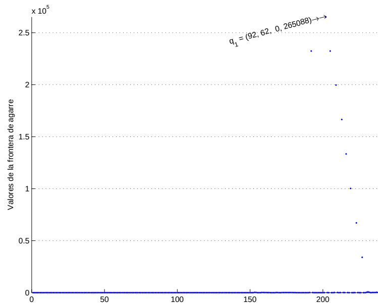
(a) Perfil de la frontera de agarre para d_h = 2 y \theta = 0
