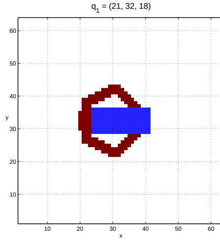
Figura 4.14: Pinza en la configuración del mejor agarre q_1(x, y, \partial_g) = (21, 32, 18) .
