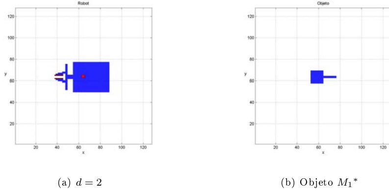
Figura 4.34: Robot con pinza con zona de agarres en la yema de los dedos y en la pieza.
