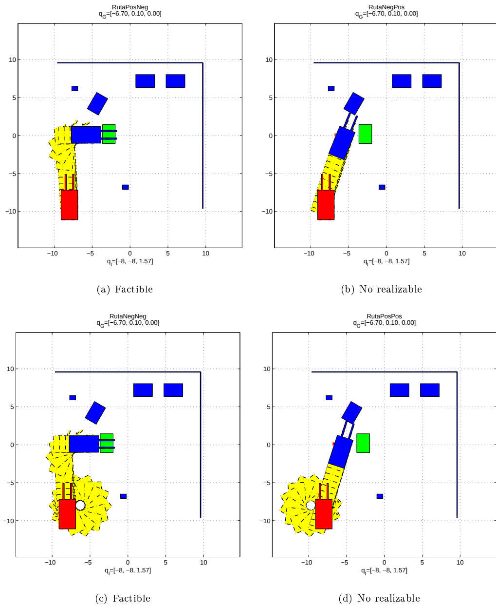
Figura 5.24: Rutas del primer grupo de configuraciones de agarre en el orden en el que han sido evaluadas. El camino de tránsito seleccionado por el planificador es el representado en (a).
