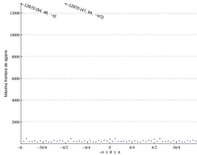
Figura 4.30: Valores máximos de la frontera de agarre en todas las orientaciones.
