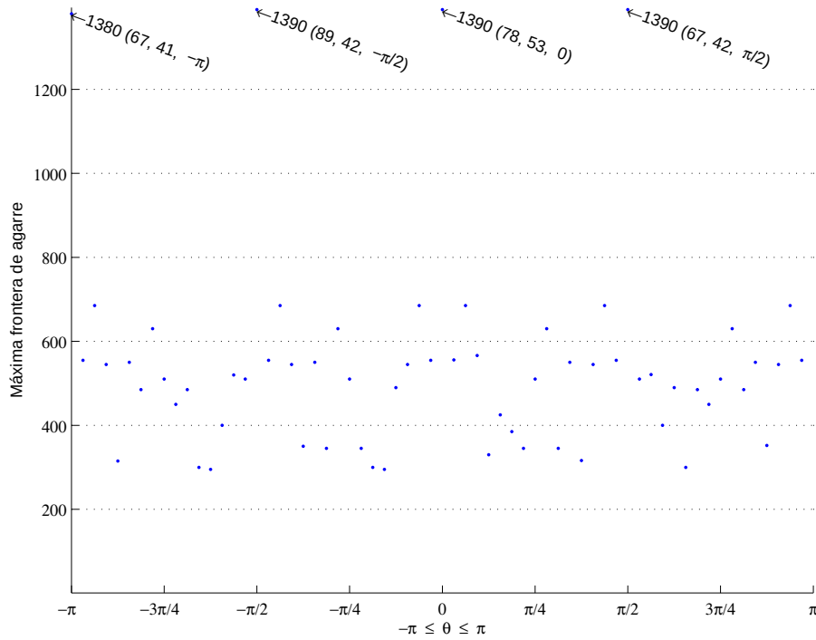
Figura 4.43: Valores máximos de la frontera de agarre en todas las orientaciones.
