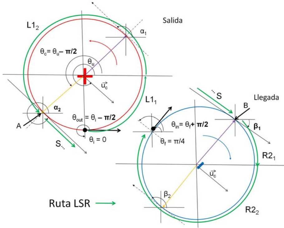
Figura 5.22: Esquema del cálculo de la curva de Dubins LSR
