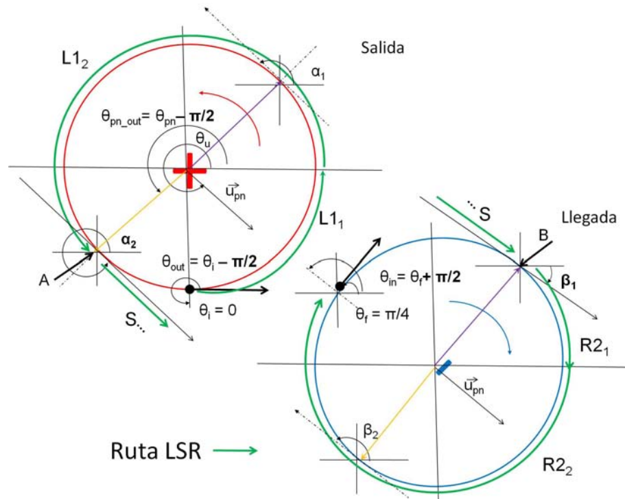
Figura A.4: Esquema del cálculo de la curva de Dubins LSR.
