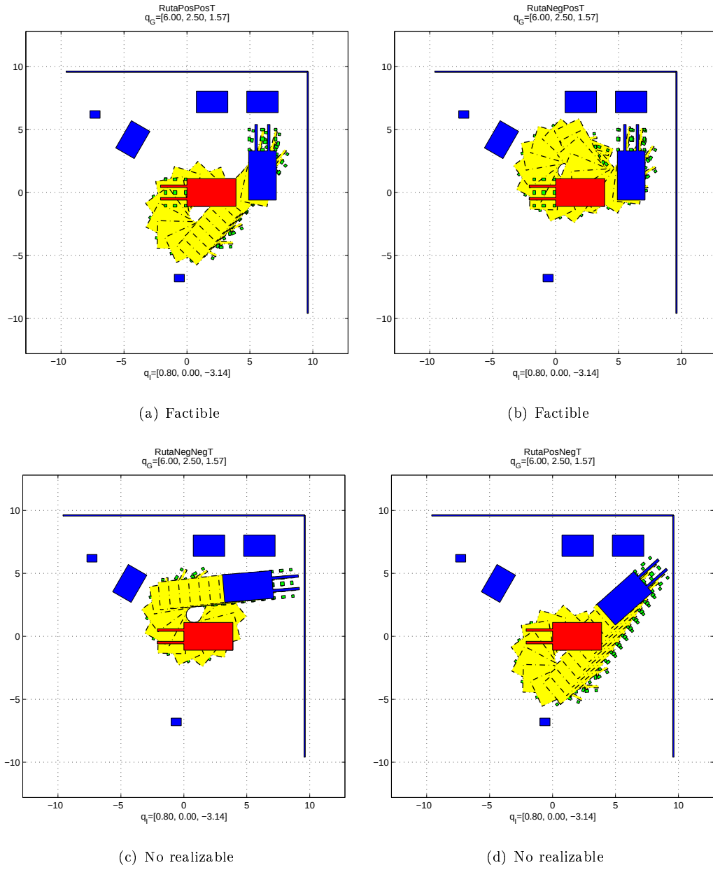
Figura 5.29: Caminos de transferencia desde el segundo grupo de agarres.
