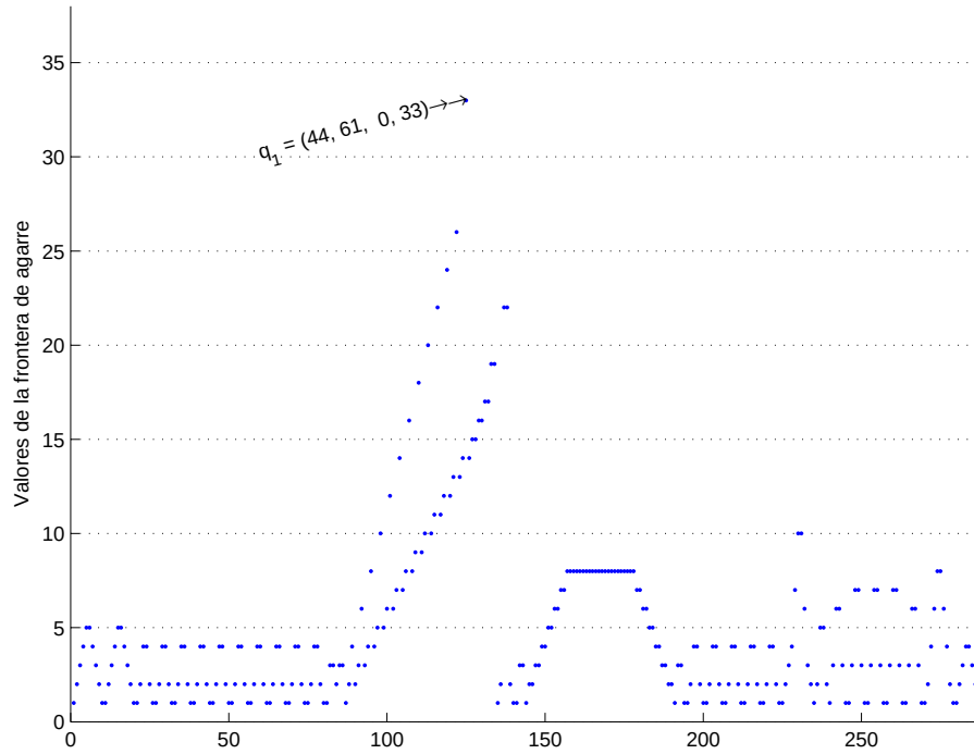
Figura 4.5: Perfil de la frontera de agarre.
