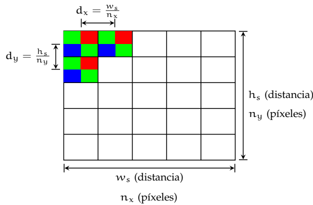
Figura 4.2.6: Dimensiones del sensor CMOS y distancia entre píxeles ( d_x, d_y ). Cada píxel se forma interpolando dos muestras de color verde, una roja y una azul mediante un filtro de Bayer.
