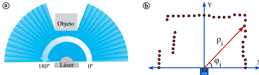
Figura 4.1.2: a) Barrido del SICK LMS 200. b) Coordenadas (\rho, \varphi) de un punto láser.
