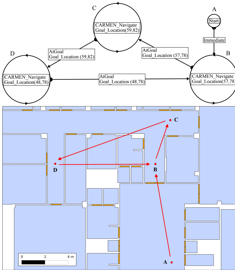
Figura 6.2.7: Misión en el interior de un departamento. La misión comienza en el punto A y a continuación define el ciclo BCDDB, que se repite indefinidamente.
