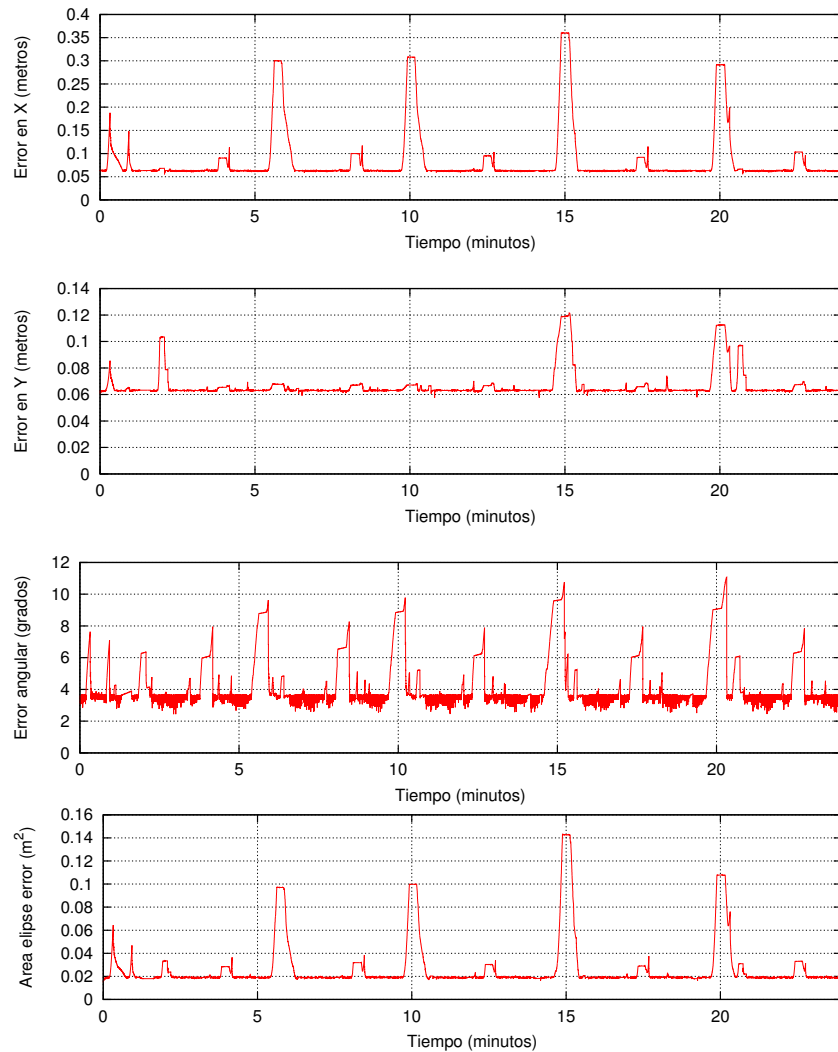
Figura 6.2.9: Errores 2\sigma_x , 2\sigma_y y 2\sigma_\theta y área de la elipse de error del 95 % durante la trayectoria estimada mediante EKF de la figura 6.2.8.
