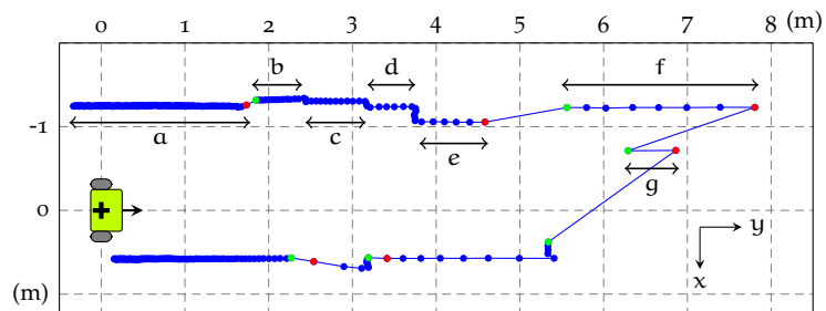
Figura 5.2.5: Etiquetado de superficies ( a - g ) para la pared izquierda. Los puntos de ruptura se indican mediante verde (inicio) y rojo (fin).
