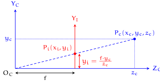
Figura 4.2.5: Proyección de un punto ( P_c ) en el plano de la imagen ( P_i ).
