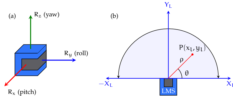
Figura 4.2.2: a) Ángulos de rotación en el láser. b) Detección de un punto en el sistema de referencia del láser.
