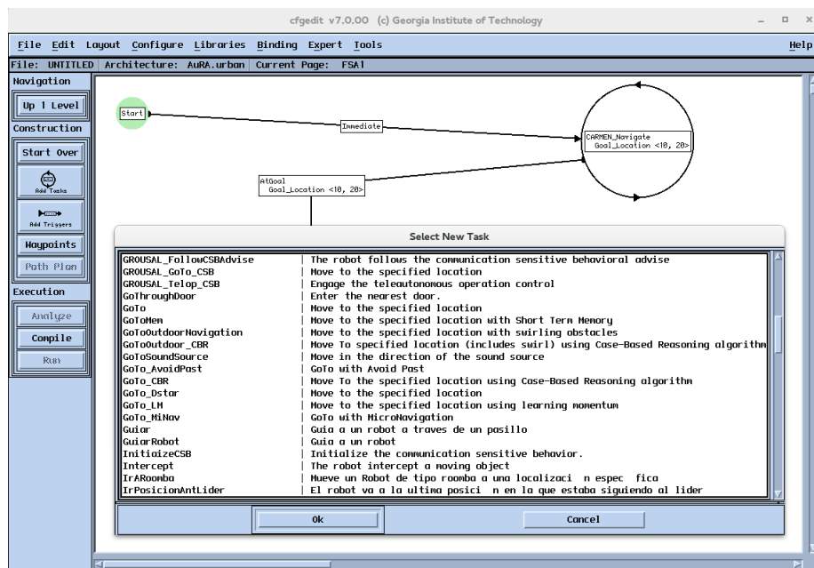
Figura 2.3: Herramienta de creación de misiones CfgEdit
