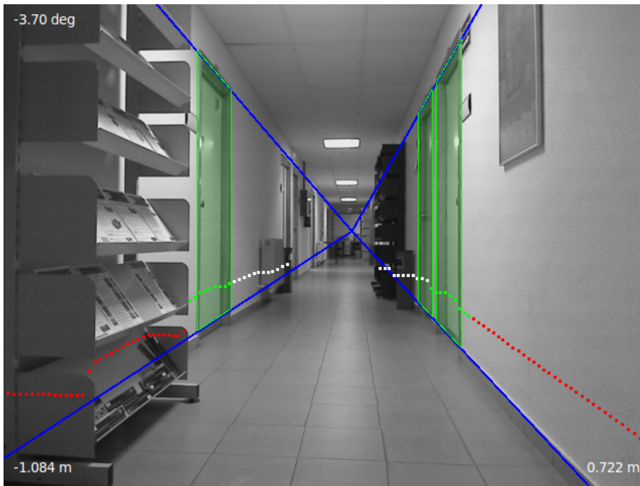
Figura 4.2: Visor del software de detección de puertas ( doorDetectionGui )
