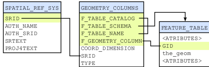
Figura 2.25: Esquema PostGIS para extender PostgreSQL con tipos geométricos
