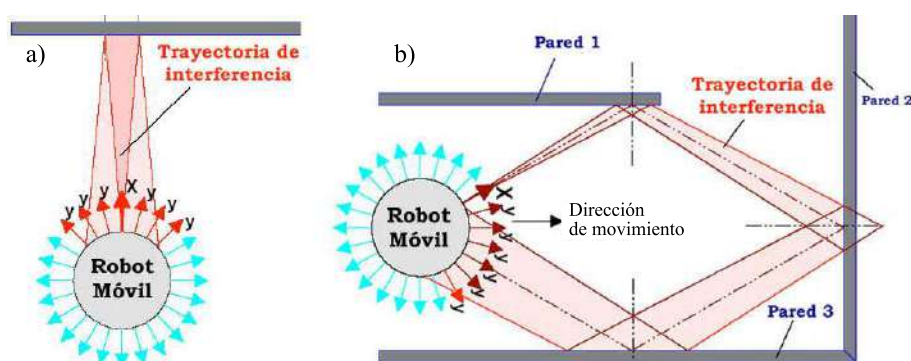
Figura 2.5: Interferencias ( crosstalk ) en el sonda: a) directa. b) indirecta.
