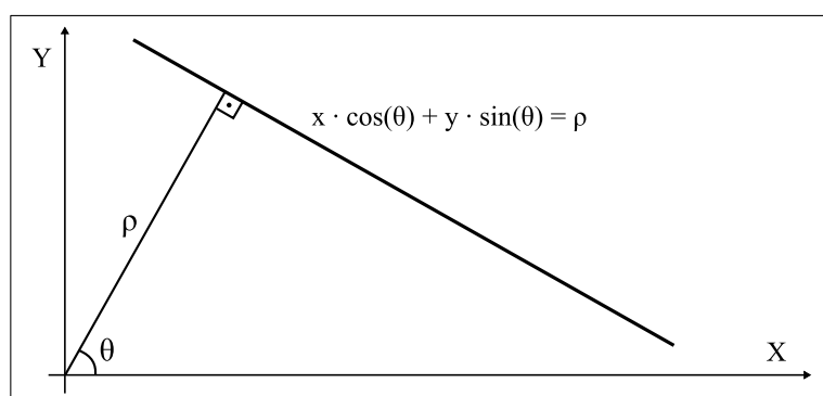
Figura 4.5: Recta en forma normal
