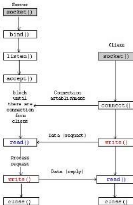
Figura 8 - Socket TCP
