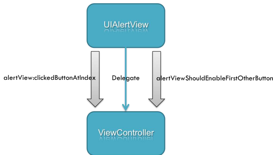
Figura 5 - Patrón Delegate
