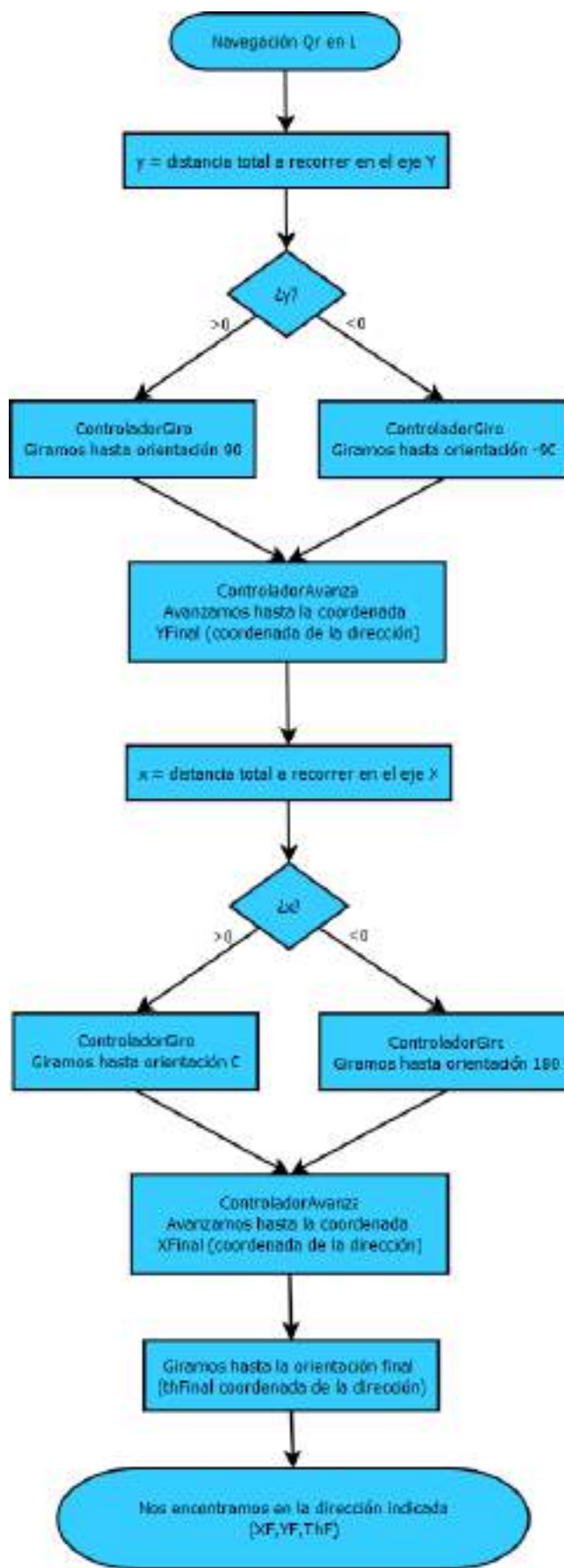
Figura 46 - Diagrama de flujo de la NavegaciónQr ServidorQrNav
