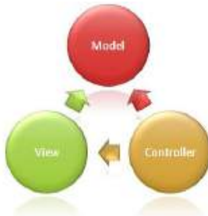
Figura 4 - Patrón MVC
