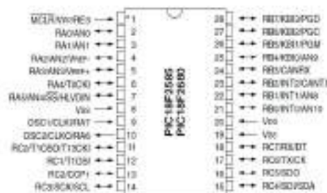
Ilustración 3: 18F2680
