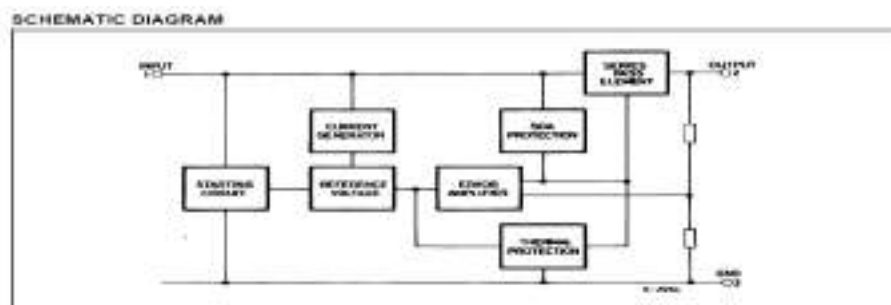
Ilustración 7: L7805CV
